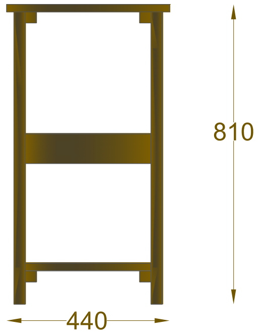
laterale
